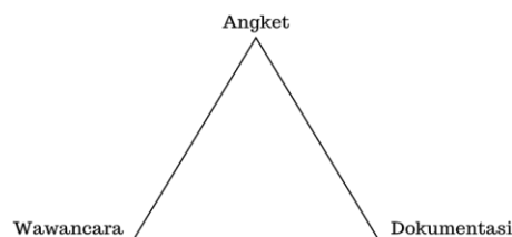
Gambar 3 : Triangulasi Sumber
